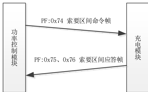
图 4 索要区间命令交互流程
