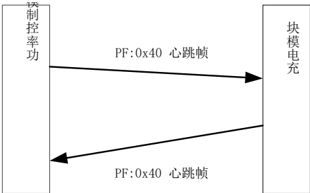
图 10 心跳帧交互流程
