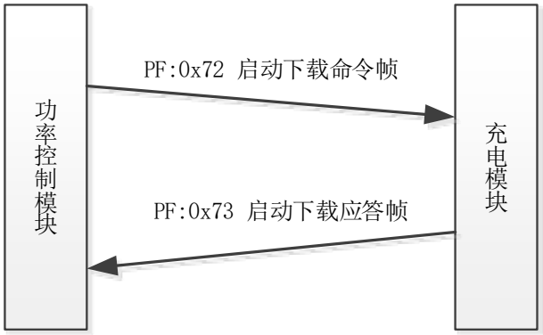
图 3 启动下载命令交互流程
