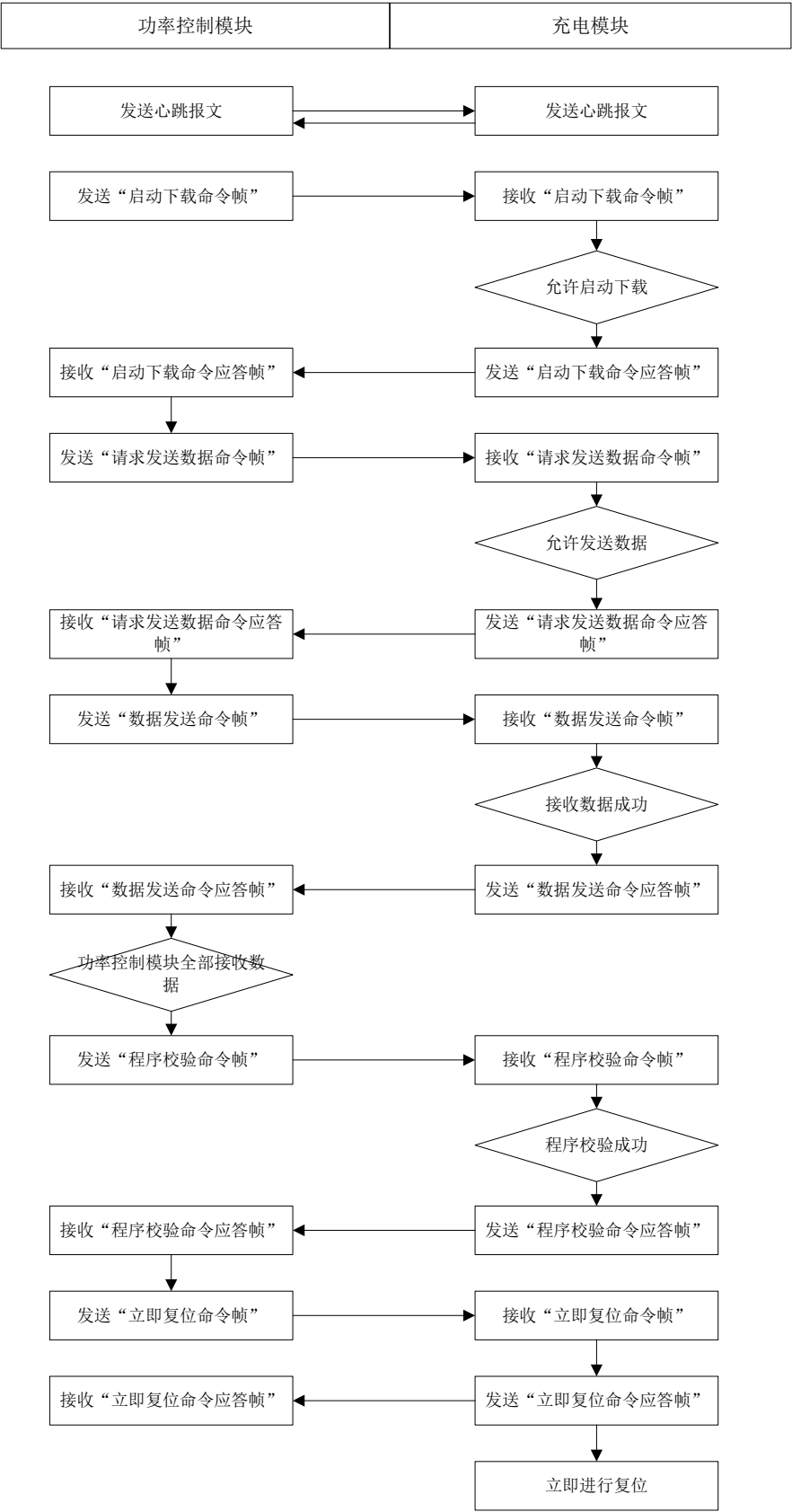
图 3 功率控制模块与充电模块程序在线更新流程图
