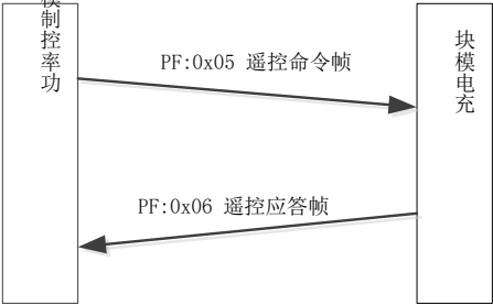
图 8 动态分组模式下遥控交互流程
