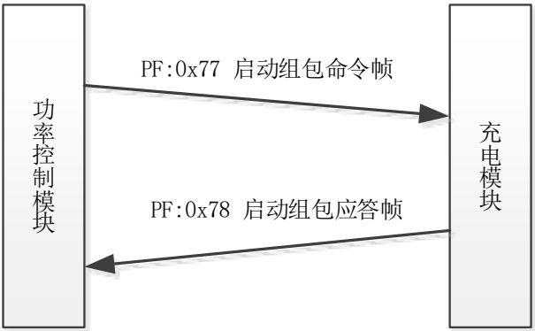
图 5 启动组包命令交互流程
